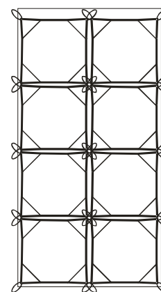
Wykorzystanie powierzchni ładunkowej przy zastosowaniu worków Q-bag
